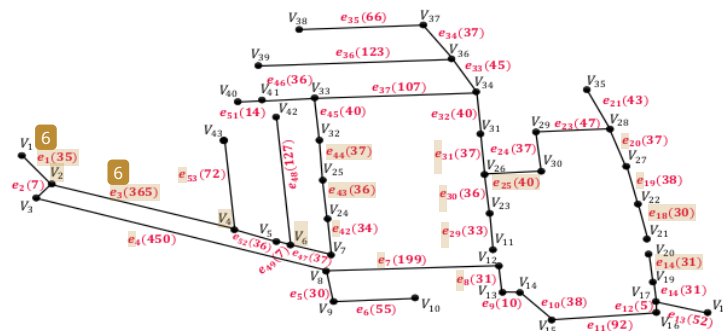
Gambar 6. Iterasi 2 Pencarian MST dengan Algoritma Kruskal
